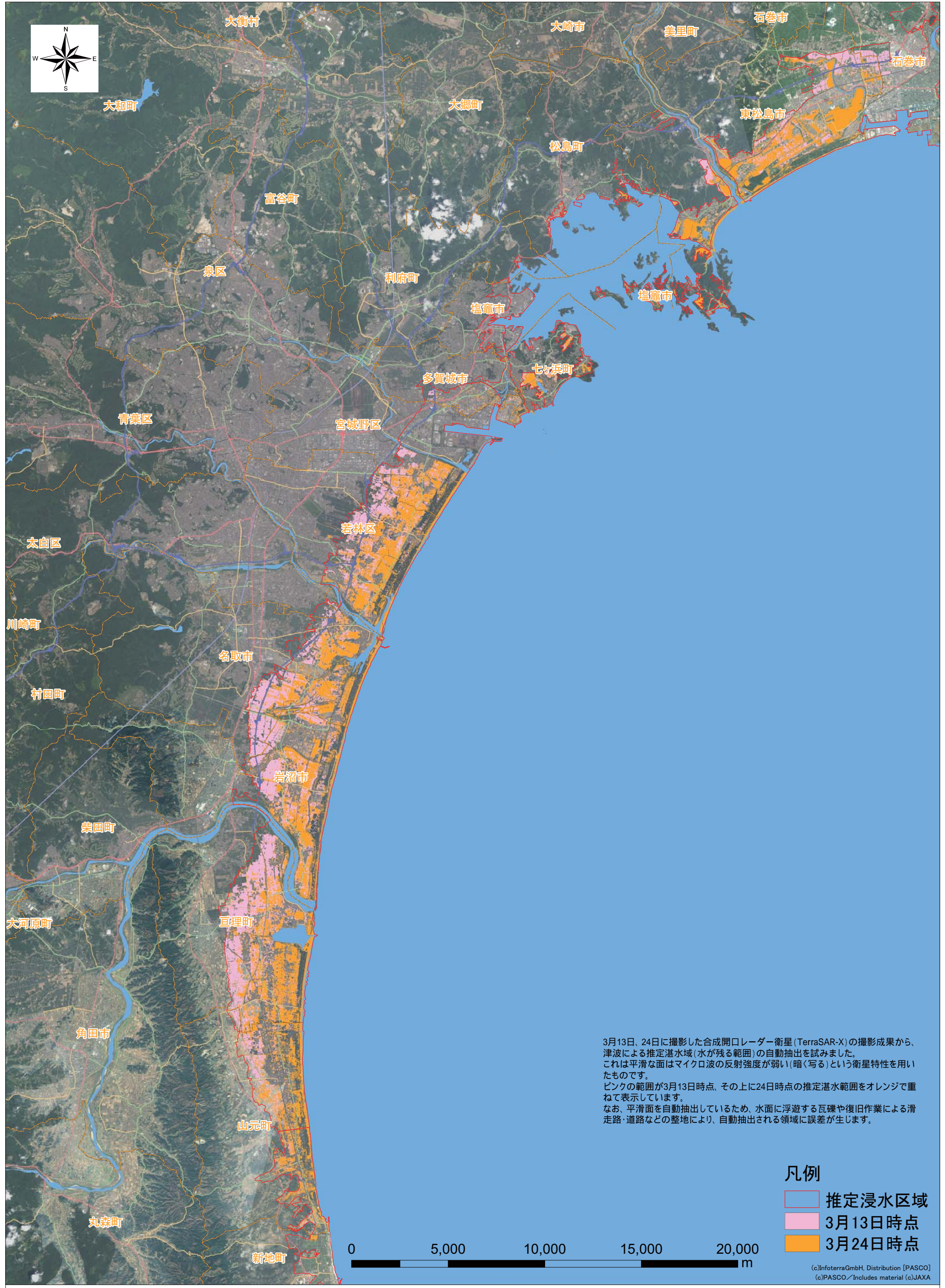
2011年3月 平成23年(2011年)東北地方太平洋沖地震 【推定】湛水域区域図(宮城県石巻市～山元町:2011年3月13日・24日)
