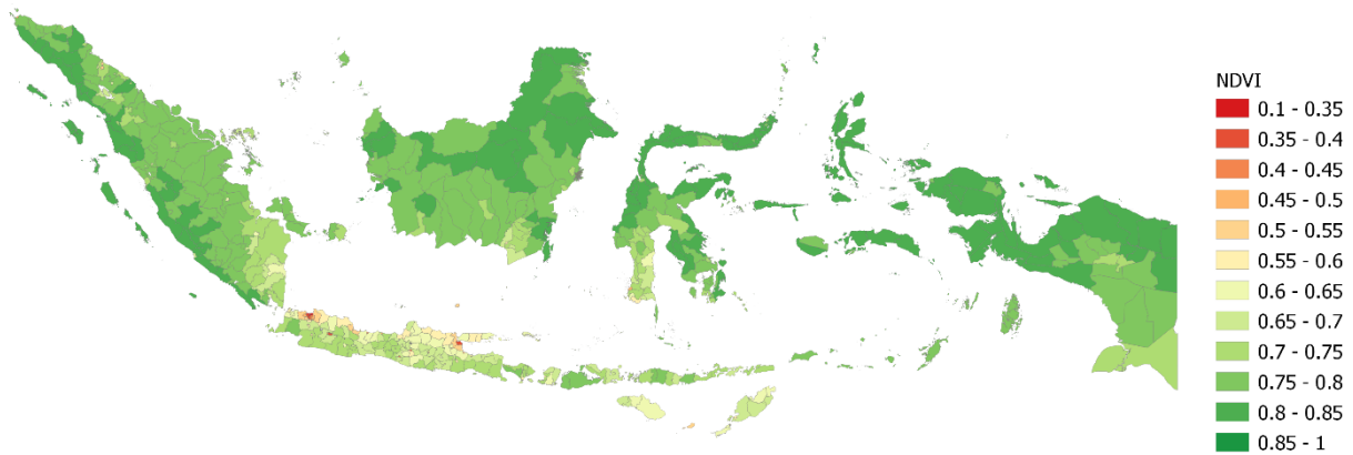
2001 年の NDVI 平均値
